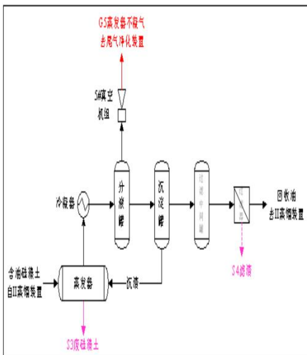
图5 高温抽提装置工艺流程图
