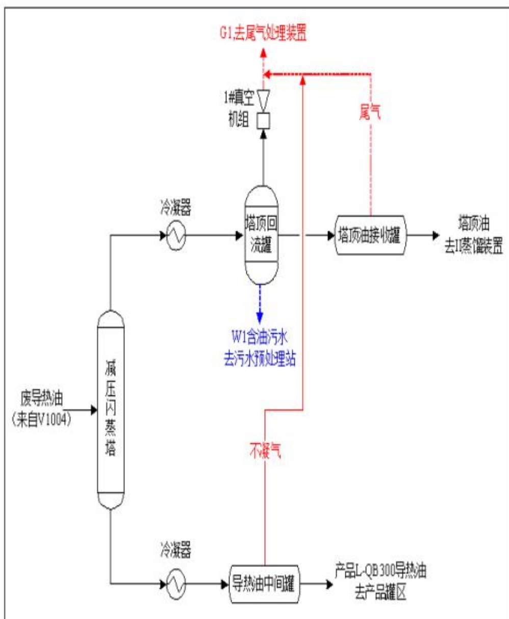
图1 闪蒸装置工艺流程图
