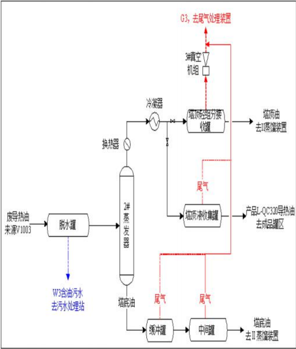
图3 I 蒸馏装置工艺流程图
