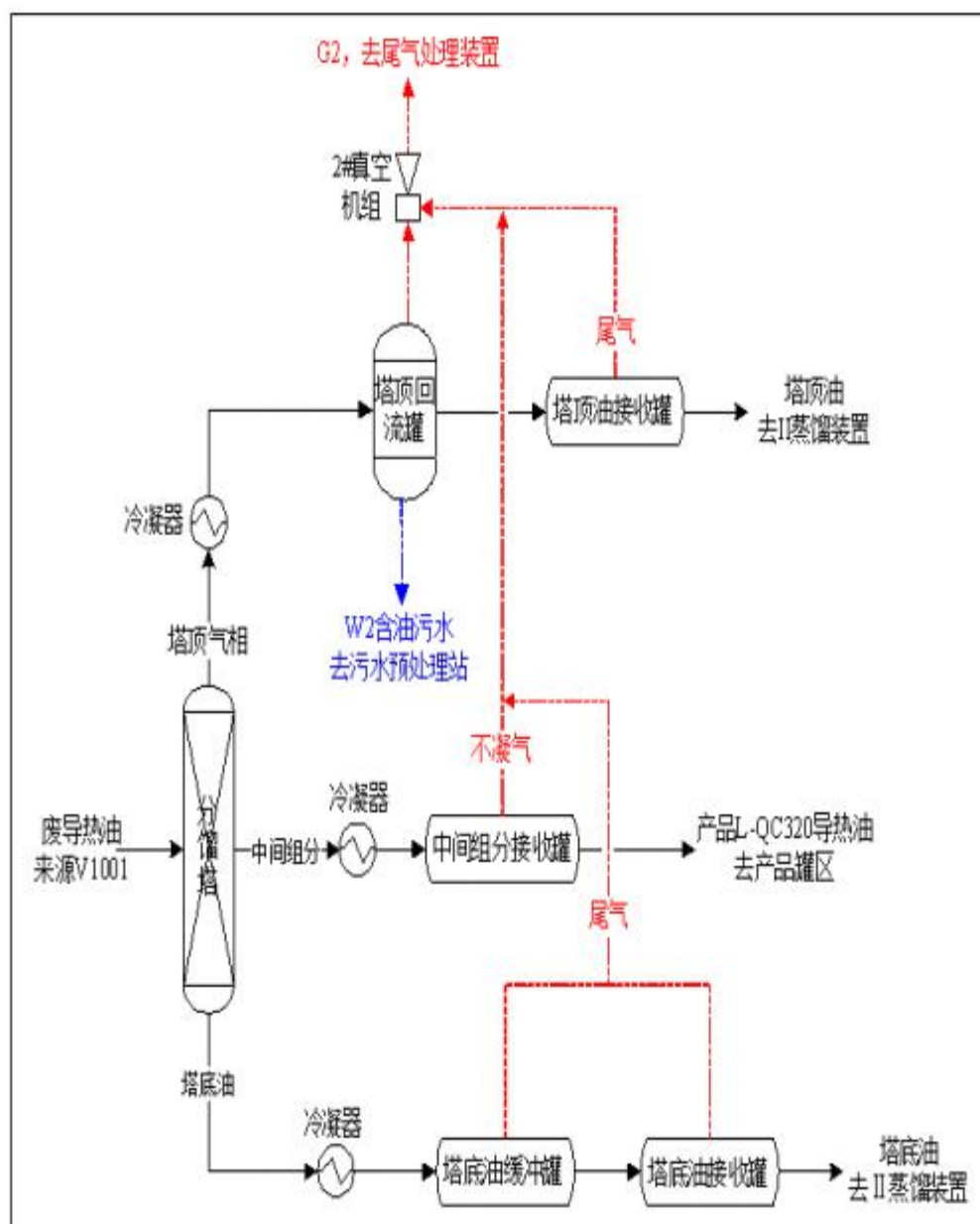
图 2 分馏装置工艺流程图
